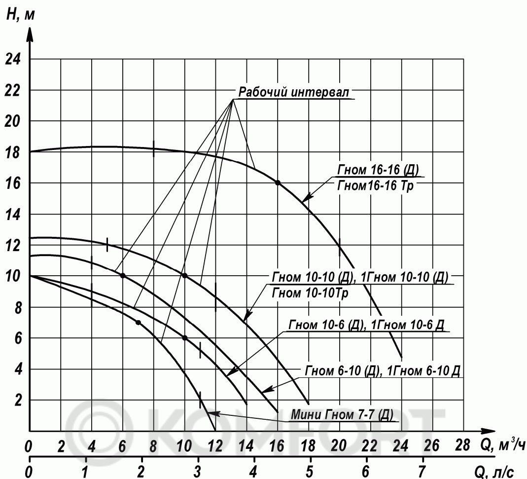
Рисунок 2 – Характеристика электронасосов
