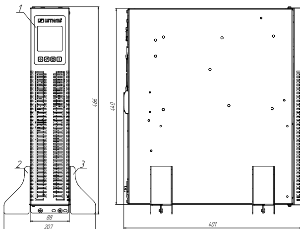
Рисунок 4б. Габаритные размеры и компоненты ИБП Штиль STR1101L, STR1101SL и STR1101LD (вертикальная напольная установка)
