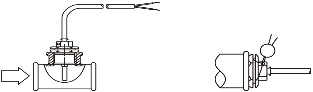
Рис. 4. Монтаж термомпреобразователя сопротивления в штуцере при помощи ниппеля и пломбирование.
