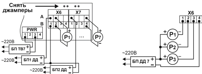
Вариант 4. Подключение ДД к ТВ7-04.1М Лайт
