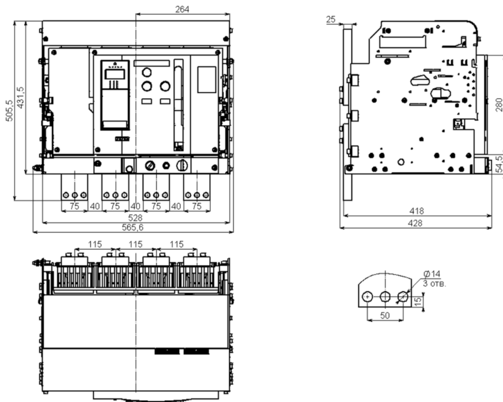
Рисунок А.20 – Автоматический выключатель YON AD-S4 выдвжного исполнения на номинальные токи 2500–3200 А переднего присоединения 4 полюса
