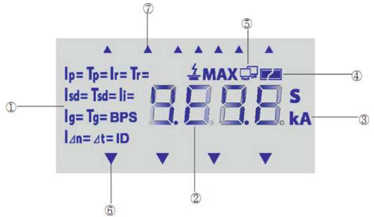
Рисунок 5 – Жидкокристаллический дисплей MR8.0
