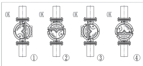
Рис. 4 Возможные положения блока управления
