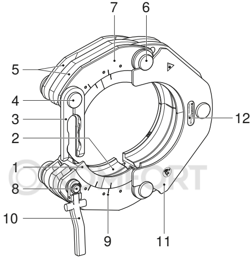
طوق كبس Geberit Mapress قطره 108 مم
