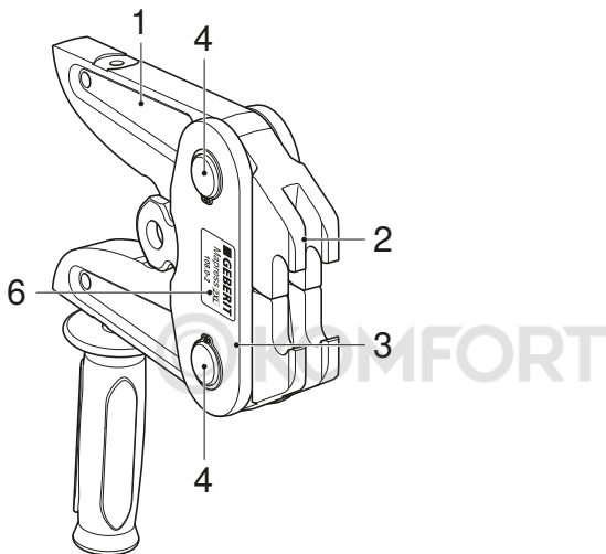
Geberit Mapress presēšanas adapters [2XL], ZB 221 un ZB 222
