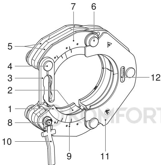
Фигура 2: Притискач клуп Geberit Mapress \varnothing 108 mm
