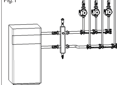
Ejemplo de instalación de un separador hidráulico con colectores FAR serie START.
