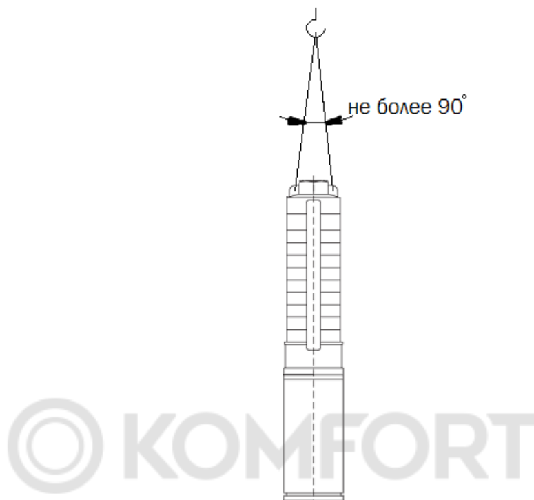
Рисунок 4 Схема строповки агрегата электронасосного
