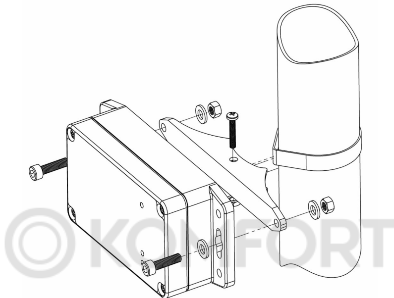
Рисунок 4 — Монтаж передающего блока на трубу
