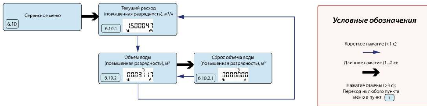
Рисунок 19 — Структура меню поверки счетчика воды
