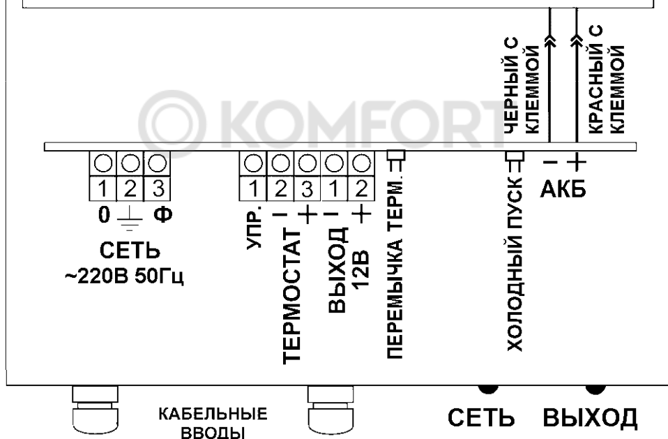
Рисунок 1 - вид изделия с открытой крышкой (схема подключения)
