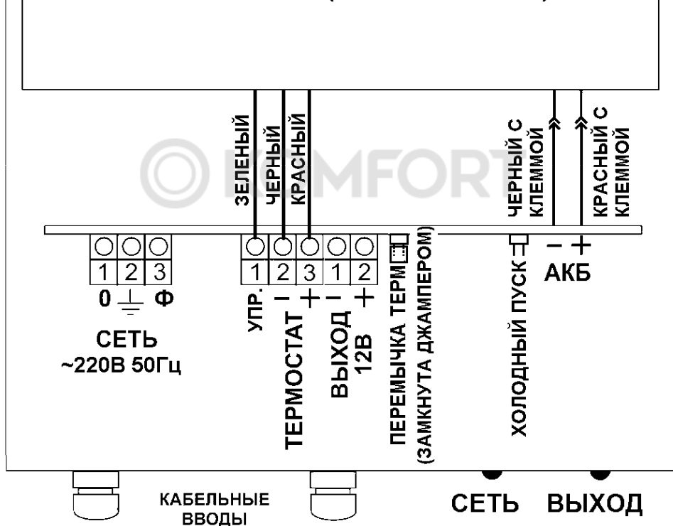
Рисунок 3. Экономичный вариант подключения термостата АКБ к изделию (с отключением термостатировани в режиме «Резерв»)
