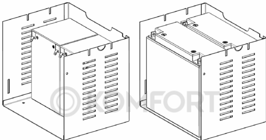
Установка двух АКБ ёмкостью 12 А*ч
