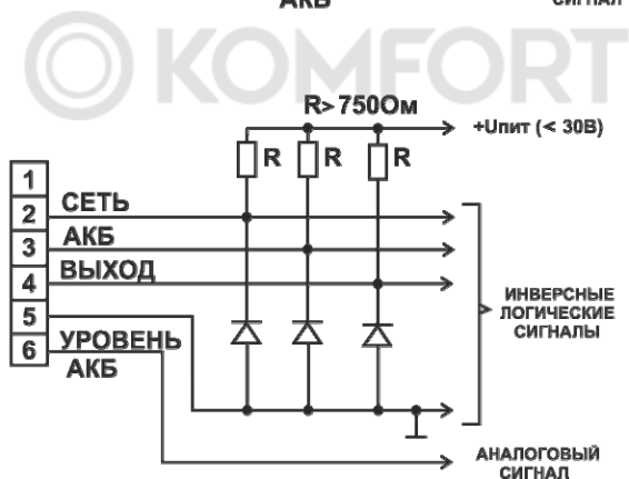
Рисунок 3. Примеры схем подключения исполнительных устройств к информационным выходам.
