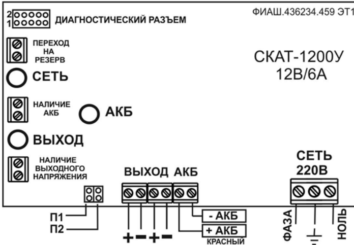
Схема подключения источника
