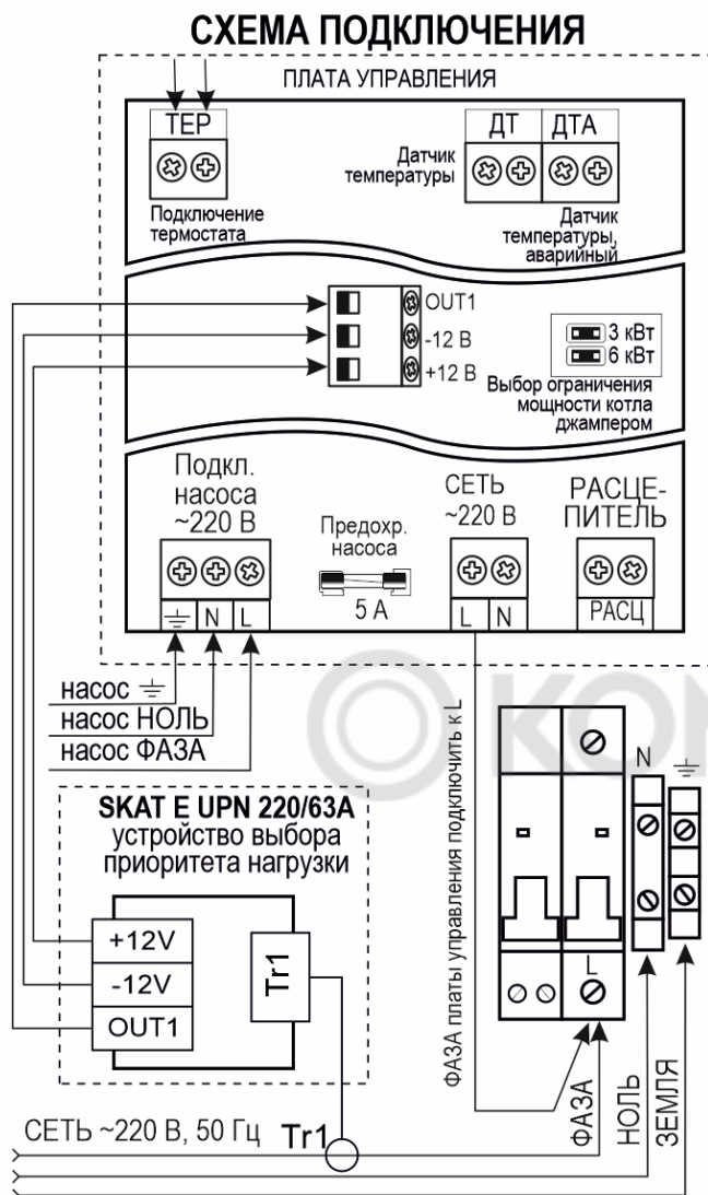
Схема подключения устройства выбора приоритета нагрузки SKAT E UPN 220/63A
