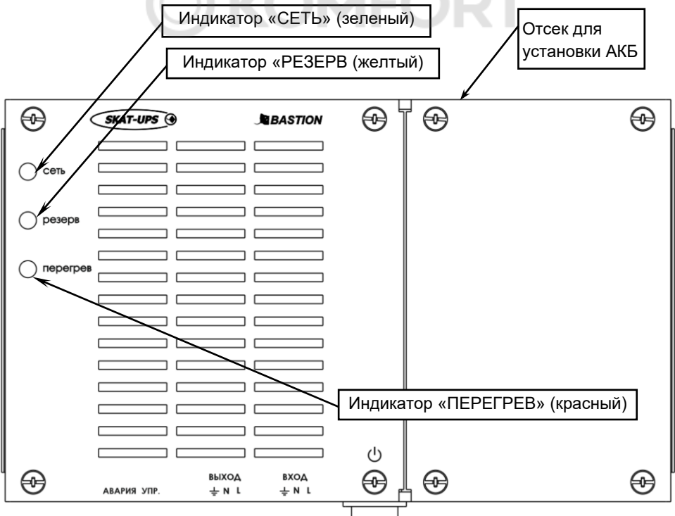
Рисунок 1 — Общий вид передней панели изделия
