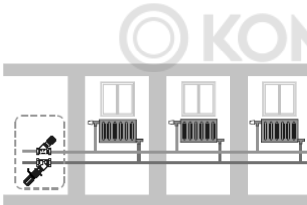
Рис. 5. Зонное регулирование с Kombi-3-plus и приводом.
