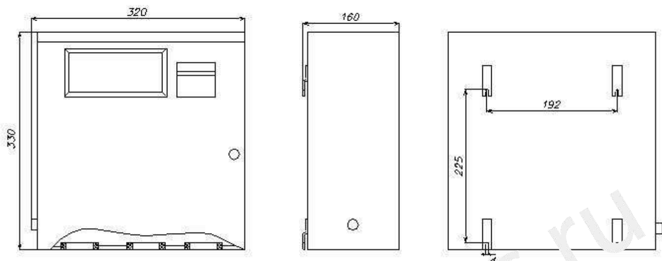
Габаритные и присоединительные размеры на станции управления СУЗ-10, СУЗ-25, СУЗ-40
