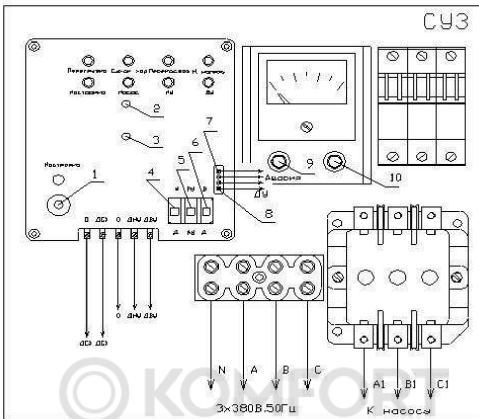
Рис. 1 Расположение и назначение органов управления и индикации.
