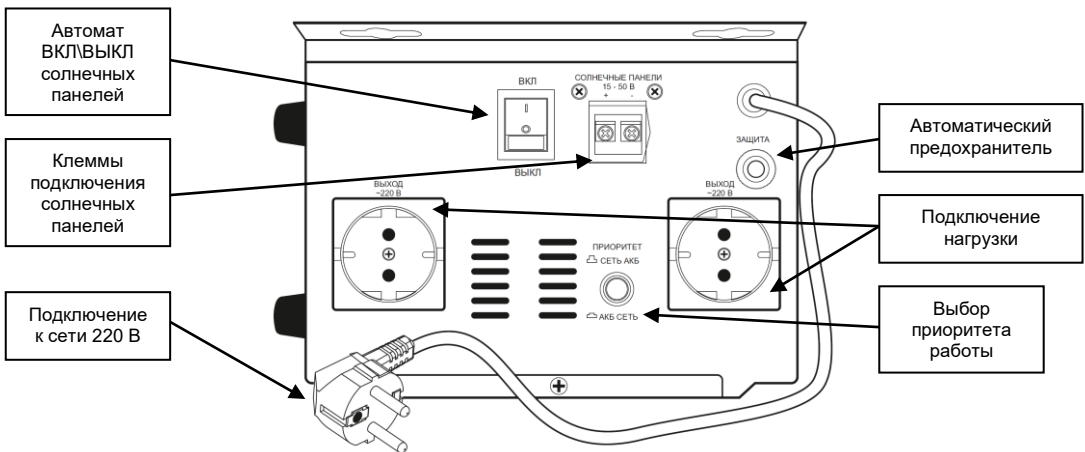
Рисунок 5 – Боковая сторона инвертора Terlocom Solar 800
