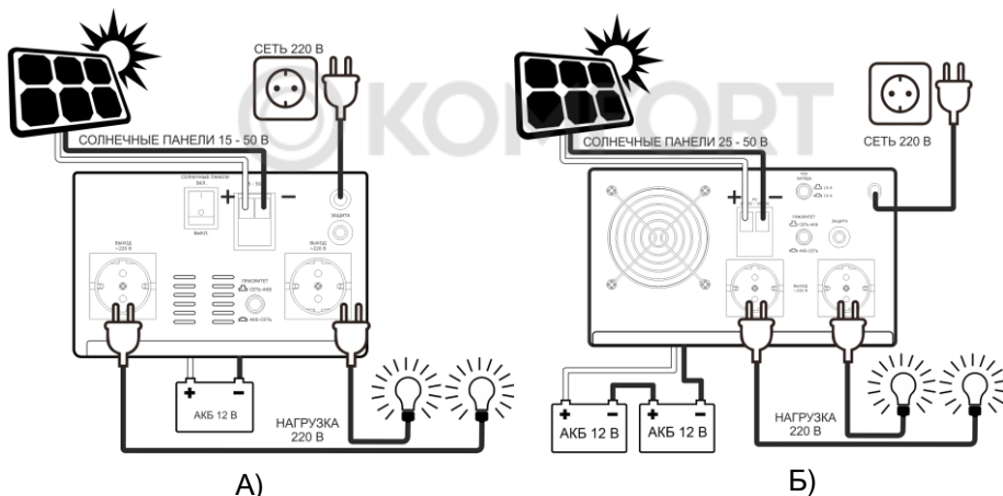
Рисунок 7 – Схема подключения: А – Теплосолар 800, Б - Теплосолар 1500.
