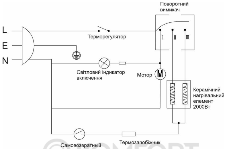
Мал.3 Електрична схема STORM 2
