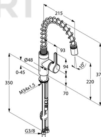
Размеры
