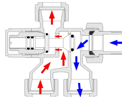
Εικ.1: Τομή διακόπτη με άξονα εντελώς ανοιχτό (μέγιστη παροχή στο σώμα και ελάχιστη στο by-pass)
