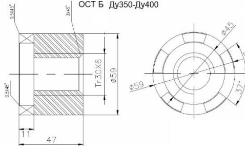
ОСТ Б Ду350-Ду400
