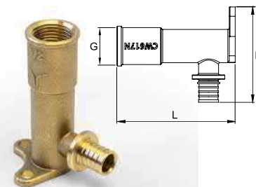
Угольник 90° с настенным креплением (водорозетка – удлиненная)
