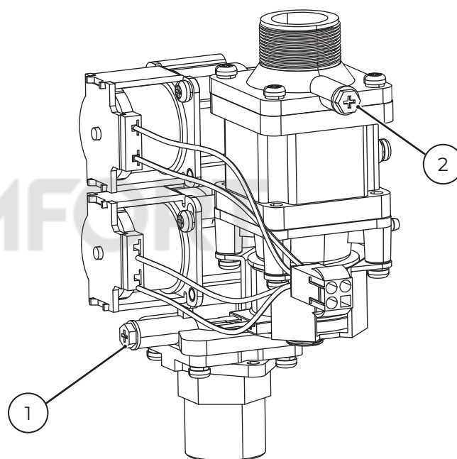
Рис. 25. Газовый клапан.
