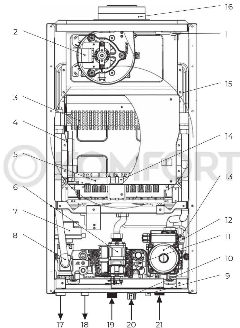
Рис. 3. Общая схема котлов B30 28 C, 32 C, 36 C.
