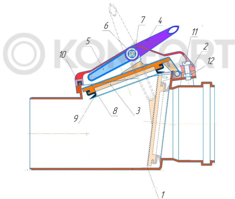
Рисунок 1. Конструкция обратного клапана
