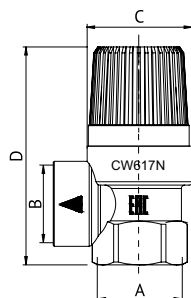
Клапан предохранительный ВВ
