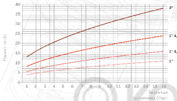
РАСХОД СПУСКА H 2 O - 1811.0-1821.0-1831.0 2"±1/2±3"
