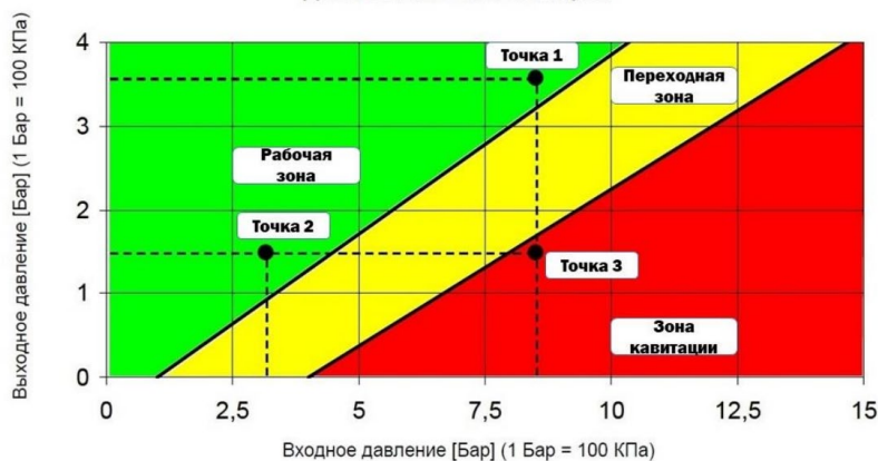
ДИАГРАММА КАВИТАЦИИ
