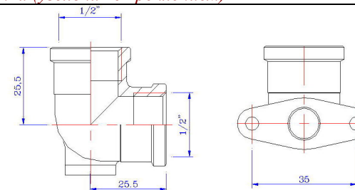
VTr. 751 Водорозетка (угольник с креплением) В-В
