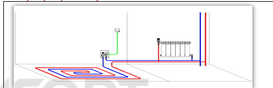
ICBOX 1.0. «Теплый пол» в высокотемпературной системе. Температура в помещении регулируется сервоприводом под управлением комнатного термостата.
