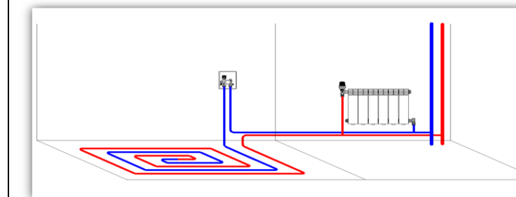
ICBOX 2.0. «Теплый пол» в высокотемпературной системе. Температура в помещении регулируется термоголовой (высота установки монтажного комплекта -1,2 м)..
