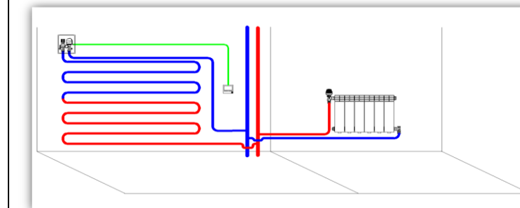
ICBOX 1.0. «Теплая стена» в высокотемпературной системе. Температура в помещении регулируется сервоприводом под управлением комнатного термостата.
