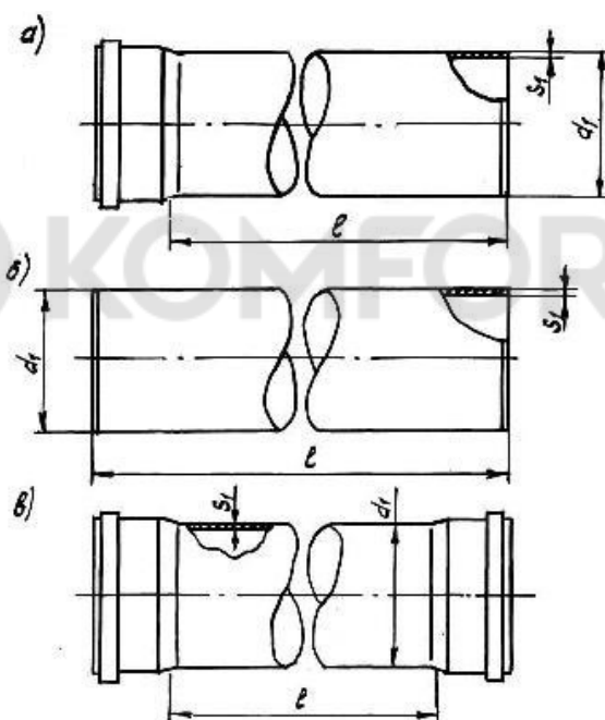
Рисунок 1. Трубы.
