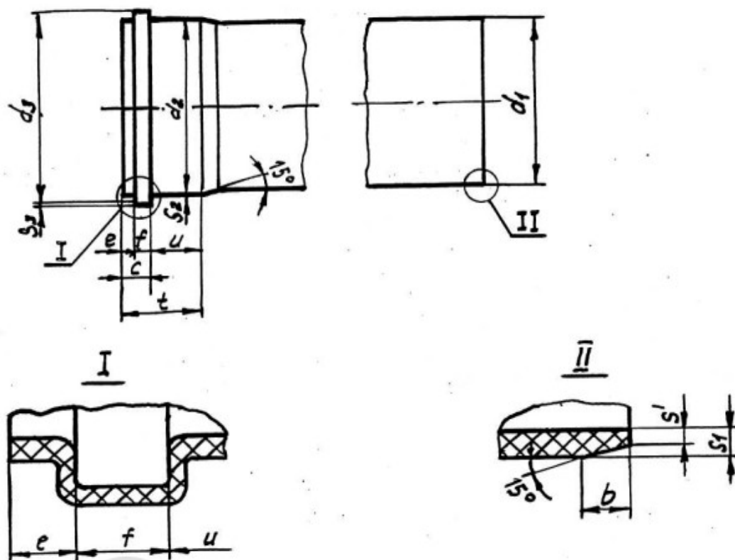
Рис. 2 Конструкция и размеры раструбных и хвостовых частей труб.
