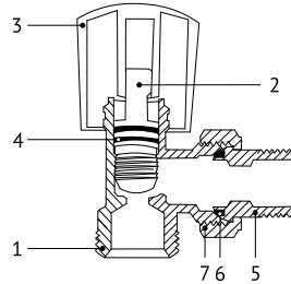
Ручной вентиль (угловой)
