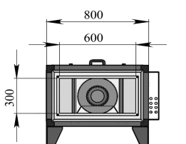
Исполнение левое Смесительный узел не показан
