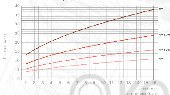
РАСХОД СПУСКА H 2 O - 1811.0-1821.0-1831.0-0111.3 2"×1 1/2"×3"
