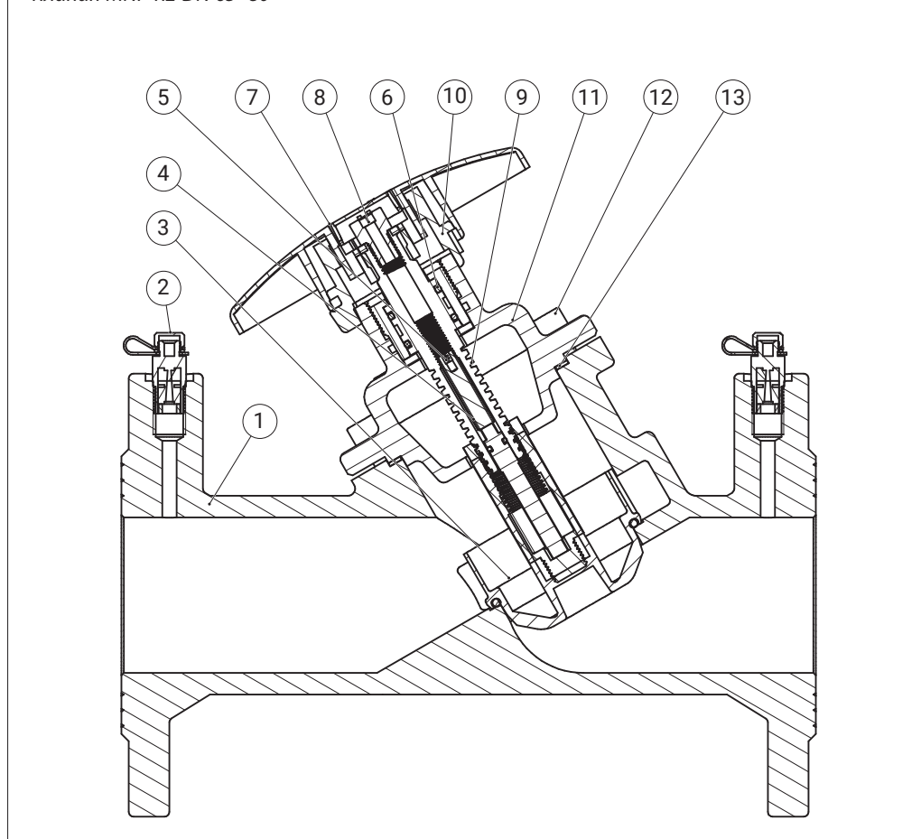
Клапан MNF-R2 DN 65–80
