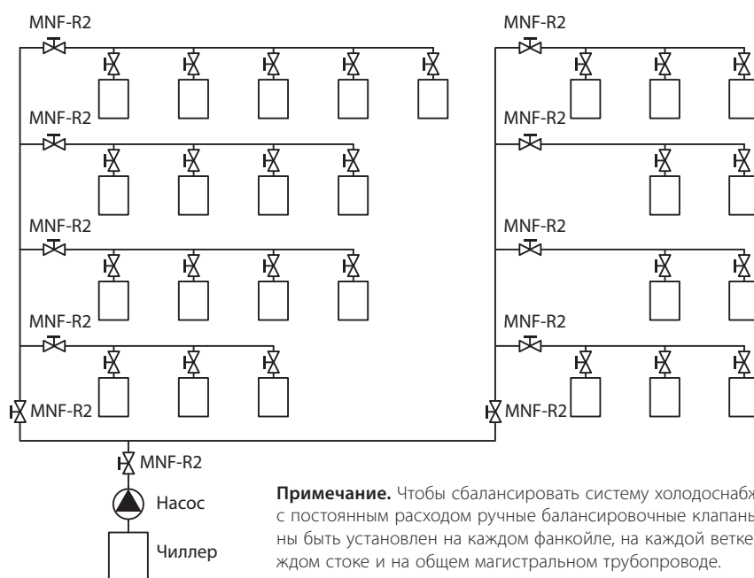
Система холодоснабжения с постоянным расходом
