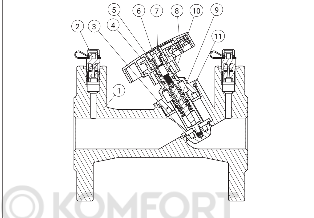
Клапан MNF-R2 DN 15–50
