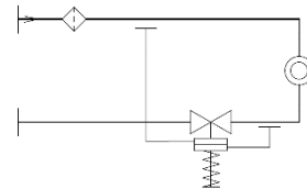
Установка регулятора на обратном трубопроводе
