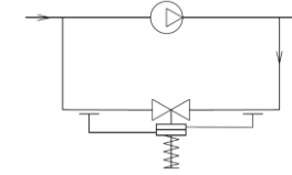
Установка регулятора на байпасе насоса
