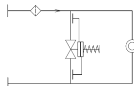
Установка регулятора на перемычке
