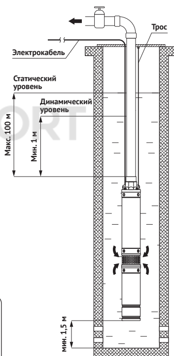
Рисунок 2 - Схема установки
