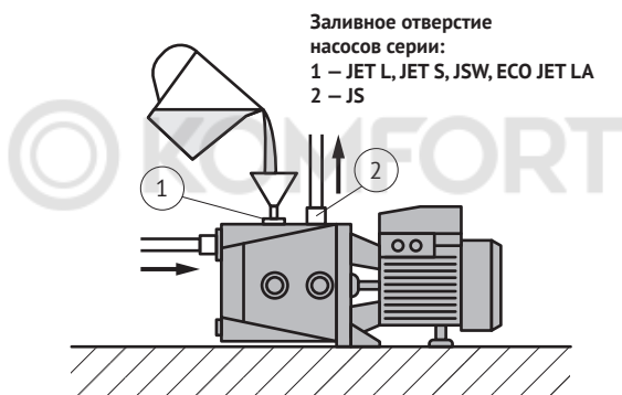
Рисунок 5 - Заполнение насоса
