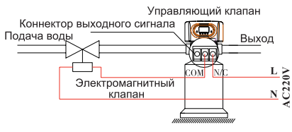
Рис. 3-2 Цепь управления электромагнитным клапаном на входе
